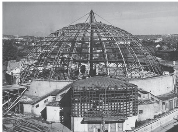
Реконструкция саратовского цирка. Конструктор В. Е. Голубинов
